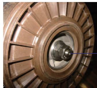
◀ Impeller
